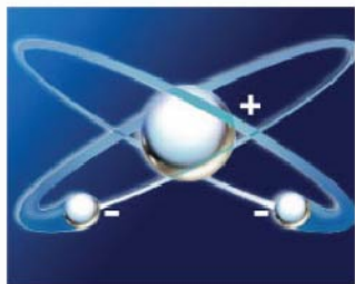
负氢离子
