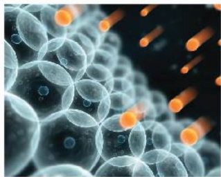
自由基
