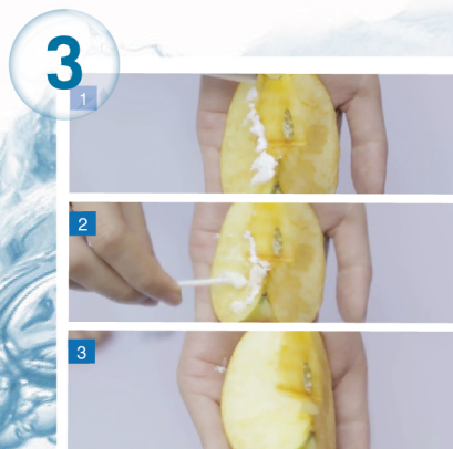
还原氧化
